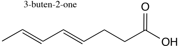
aicdo 4,6-octadienoico
