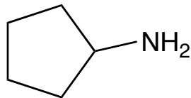
ciclopentanamina
