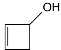
2-ciclobutenol
