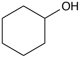
cicloesano
