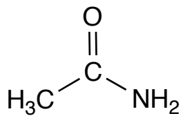
etanammide
